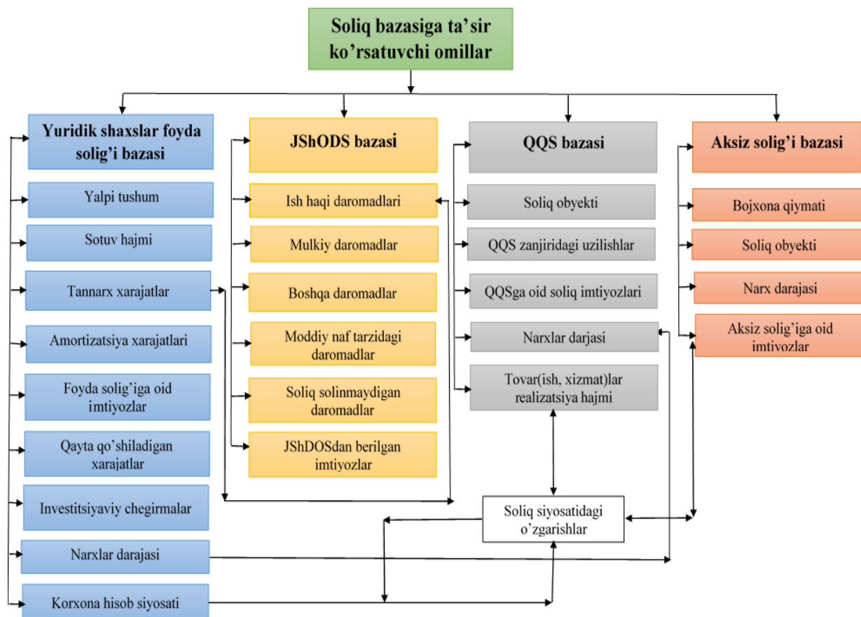
2-rasm. Soliq bazasiga ta'sir ko'rsatuvchi omillarning tarkibi 25
