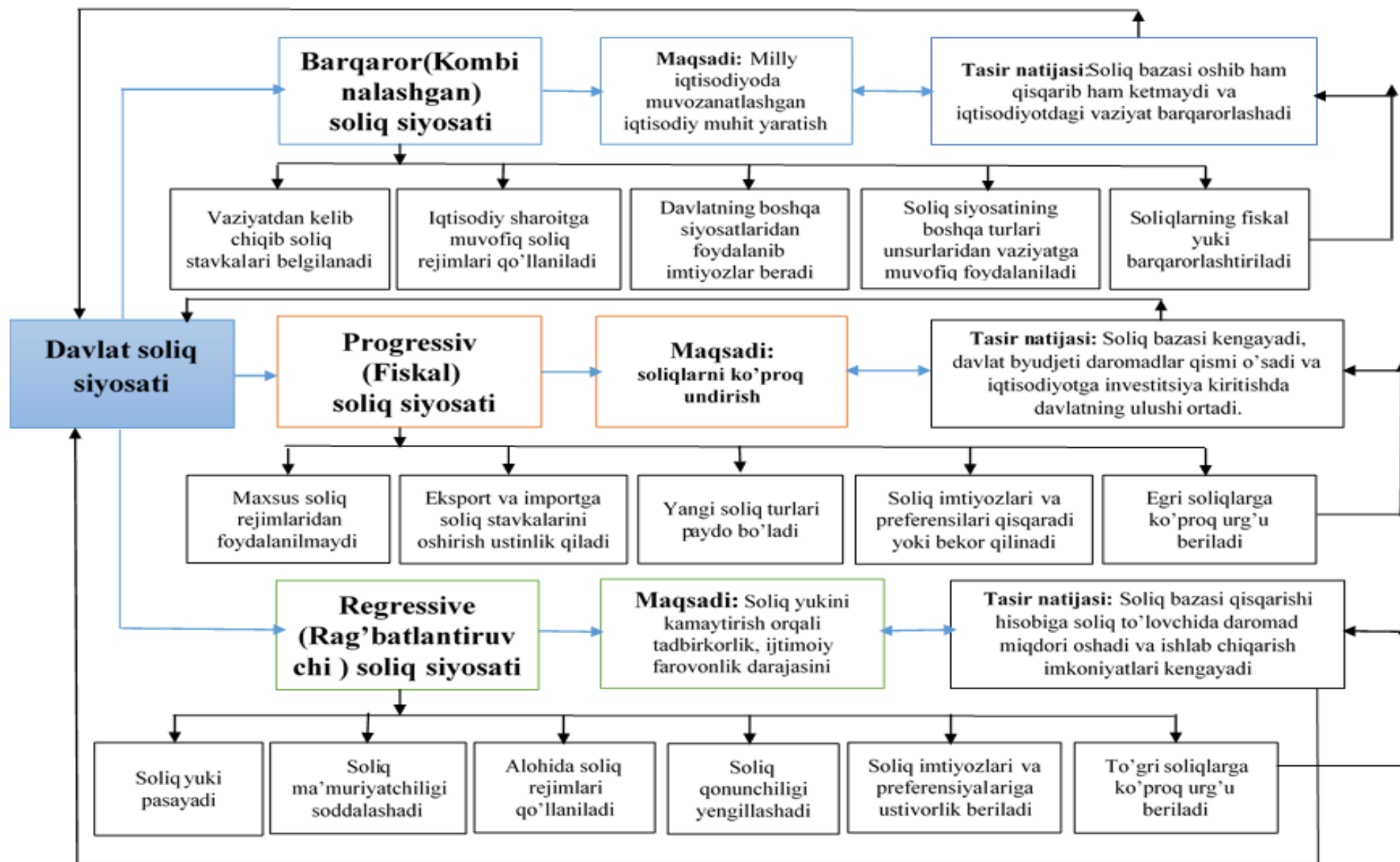
3-rasm. Soliq siyosatining soliq bazasiga ta'sirini baholashning ierarxiyal tahlili 26
