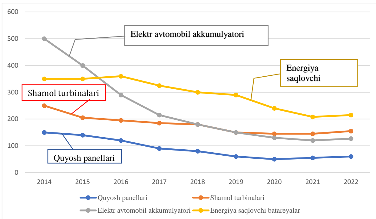
1-rasm. Yashil texnologi narxlari AQSH dollari/kVt soat (nominal narxlar) 85
