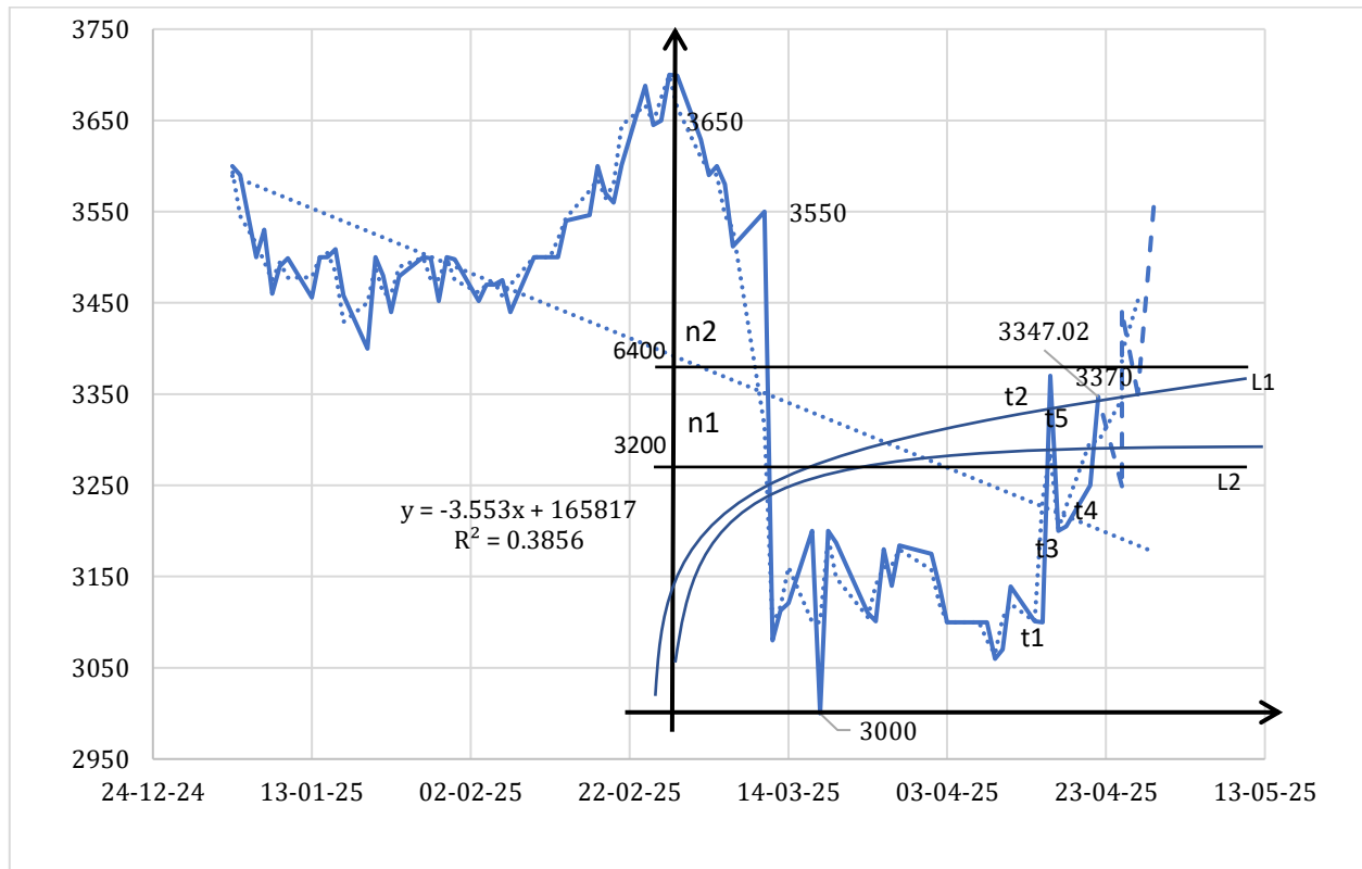
8-rasm. “O‘zbekiston respublika tovar-xomashyo birjasi” aksiyadorlik jamiyatini aksiyalar narxini o‘zgarishini Lejandra ko‘phadi funksiyalaridan foydalangan holda orqali prognoz qilish usuli
